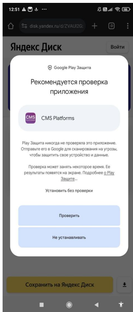
Рисунок 7 – Установка приложения
