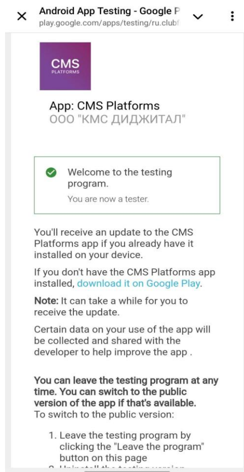
Рисунок 2 – Описание программы
